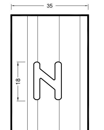
PARTICOLARE ASOLA
