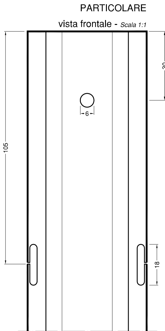
PARTICOLARE ASOLA
